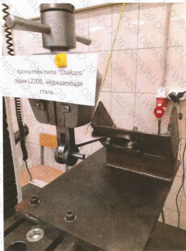
Рис. 6. Образец в процессе испытания. Схема нагружения ( F_y )
