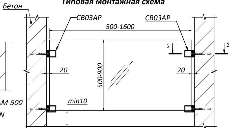
Типовая монтажная схема
