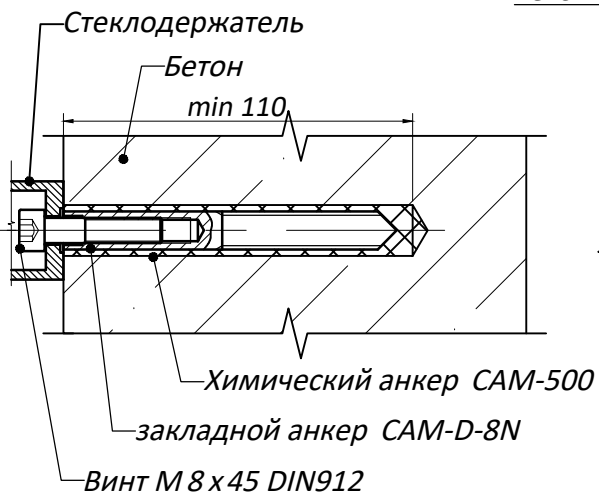
Разрез 2-2
