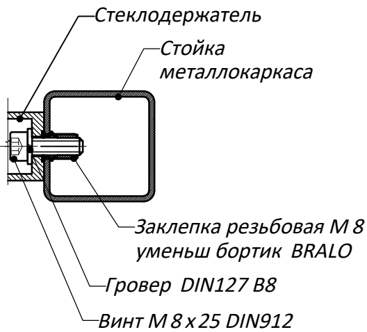
Разрез 2-2
