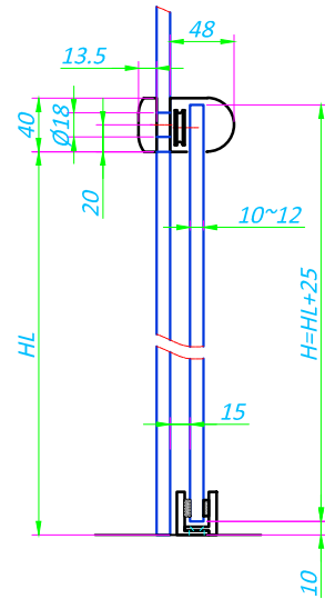
Разрез Вертикальный (5:1)
