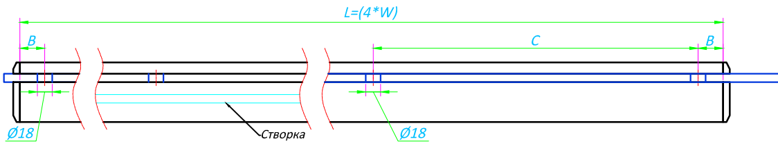
Разрез Горизонтальный (5:1)
