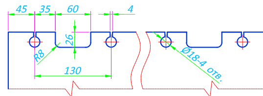
Схема отверстий в створке (5:1)
