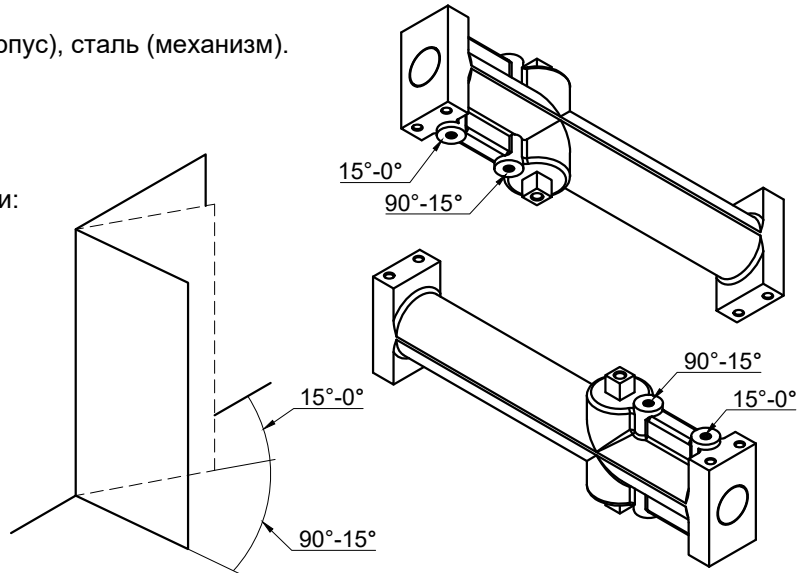
Схема регулировки доводчика
