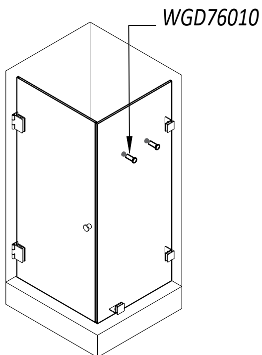
Типовая монтажная схема
