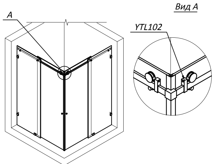
Типовая монтажная схема
