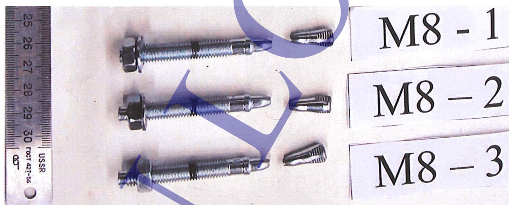
Рисунок 3. Образцы после испытания
