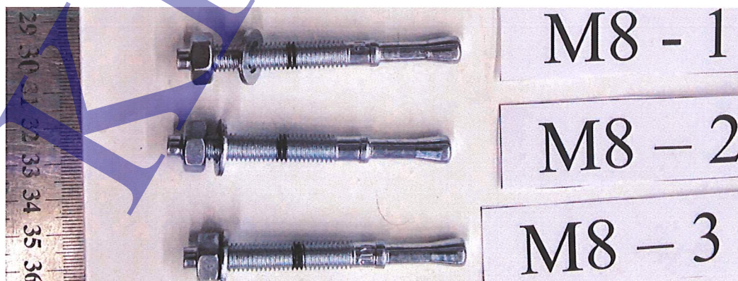
Рисунок 1. Образцы до испытания
