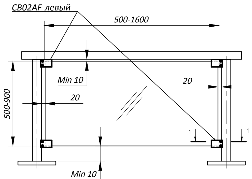
Типовая монтажная схема
