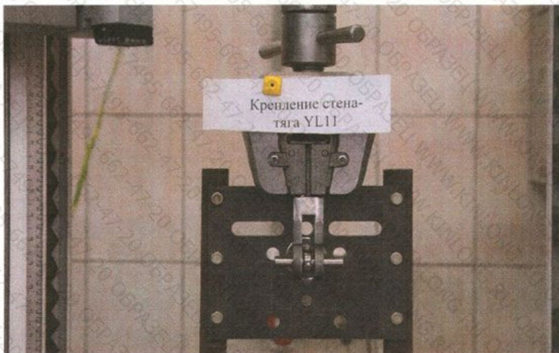
Рис. 6. Образец в процессе испытания. Схема нагружения ( F_y )
