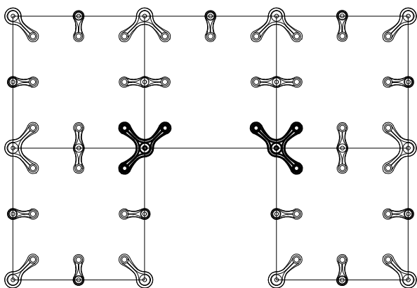
Типовая монтажная схема
