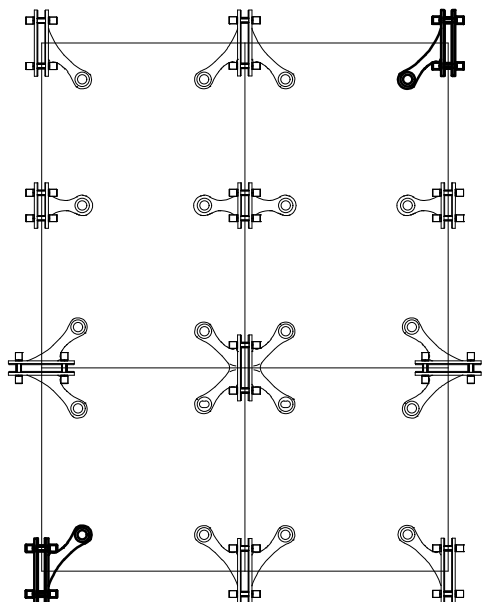
Типовая монтажная схема
