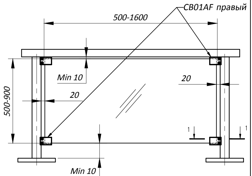
Типовая монтажная схема
